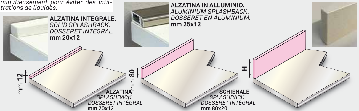
TIPOLOGIE DI ALZATINE / TYPES OF SPLASHBACK / TYPOLOGIES DE DOSSERETS
