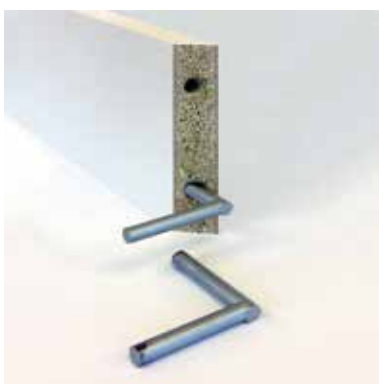
FISSAGGIO INVISIBILE PER UNIONI A 45° / INVISIBLE FIXING FOR 45° JOINTS / FIXATION INVISIBLE POUR RACCORDS À 45°
